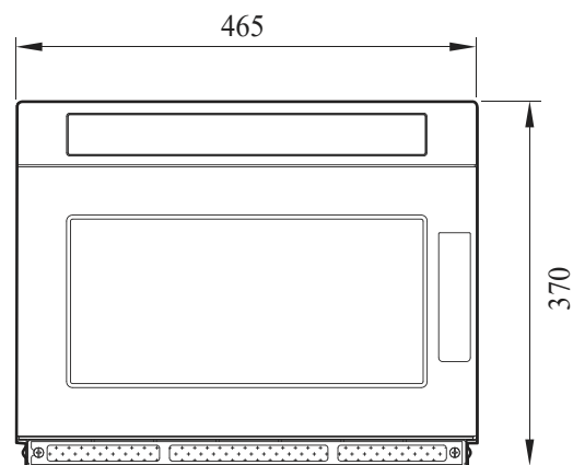
ВИД СПЕРЕДИ
